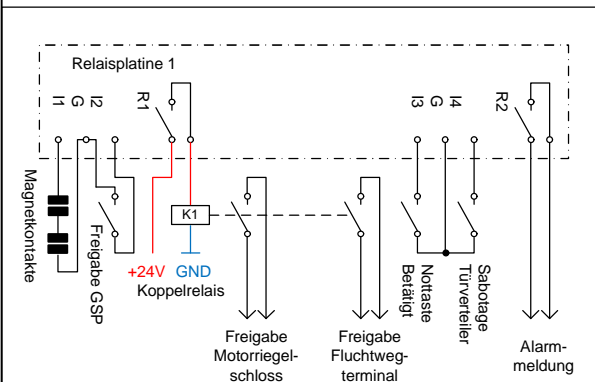
Kontaktverschaltung im Türverteiler
